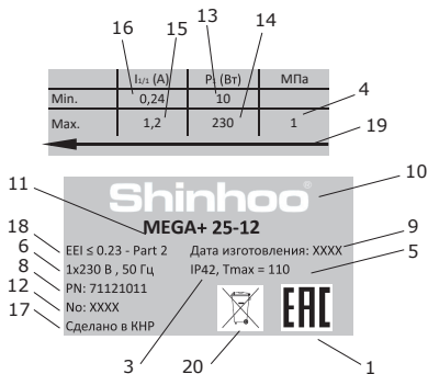
Рис. 2 Фирменная табличка насоса MEGA+
